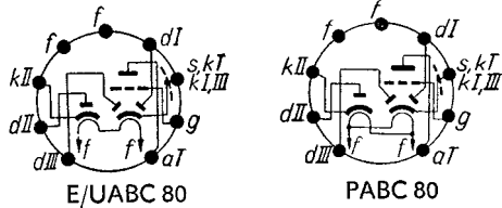
Sockelschaltenschema
