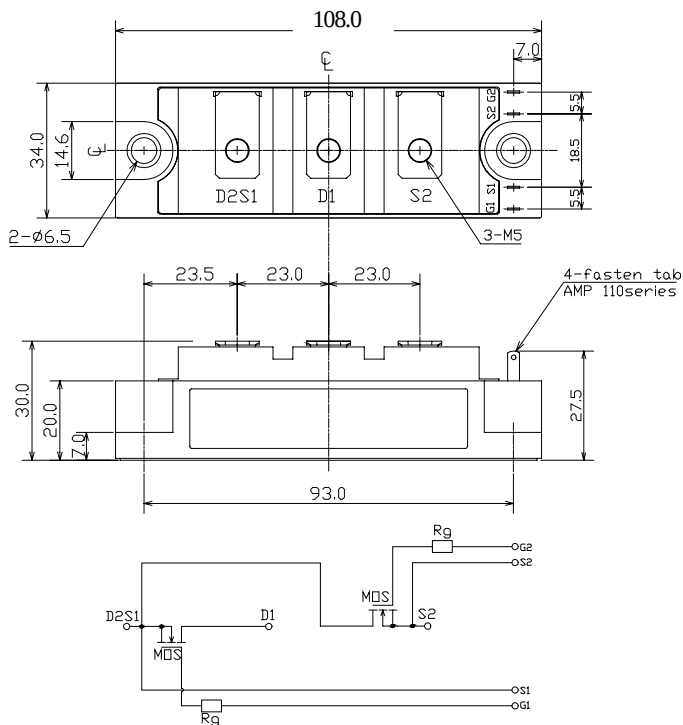
PD4M441L/440L
