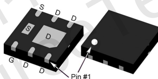
UDFN2x2-6L
