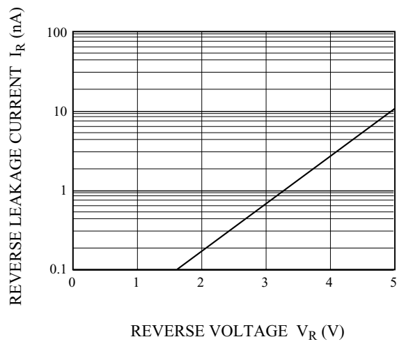
I_R - V_R
