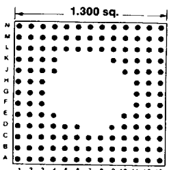
133 PINS Footprint 13048
