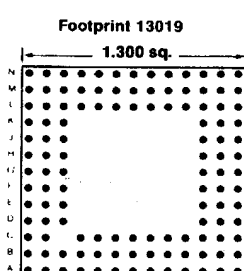
119 PINS
