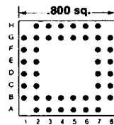
44 PINS Footprint 08003
