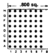
56 PINS Footprint 08004
