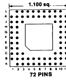
Footprint 11026
