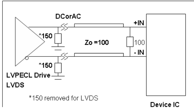
LVPECL/ LVDS Input
