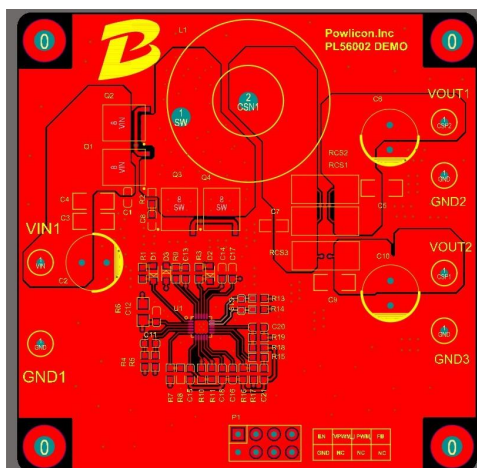
Fig. 32 Top lay
