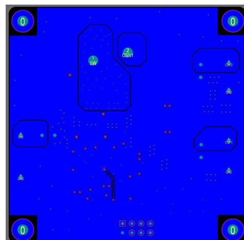
Fig. 33 Bottom lay
