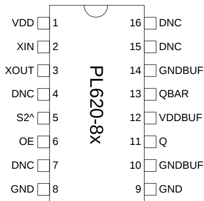
TSSOP-16L
