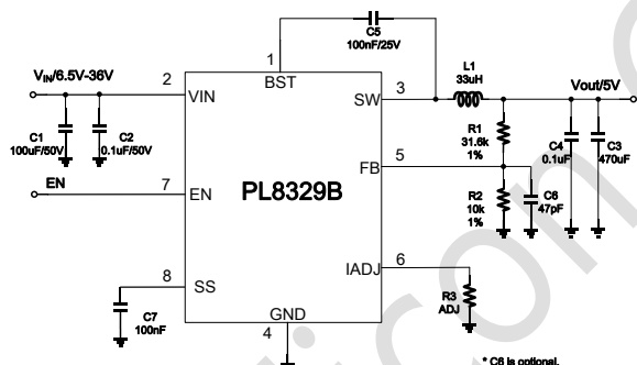
Fig. 1 Schematic
