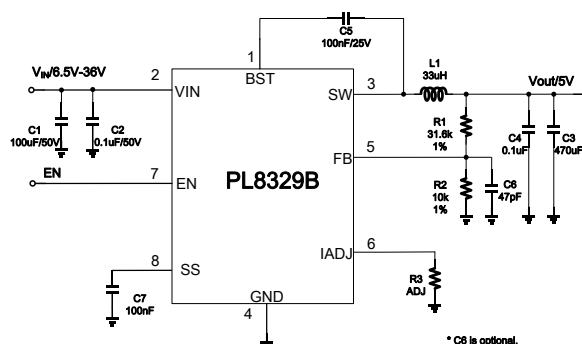
Fig. 22 Schematic
