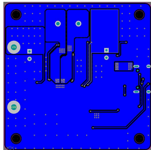
Fig. 34 Bottom lay
