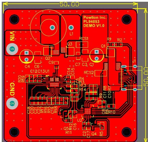
Fig. 33 Top lay
