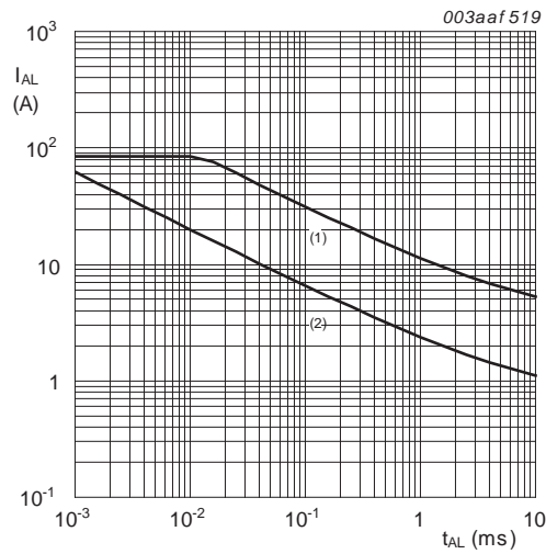
(1) T_{j(rit)} = 25^\circ C ; (2) T_{j(rit)} = 100^\circ C
