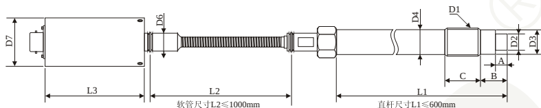
PT127系列 外型尺寸图
