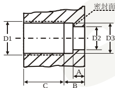
PT127系列 平端面密封安装孔尺寸图
