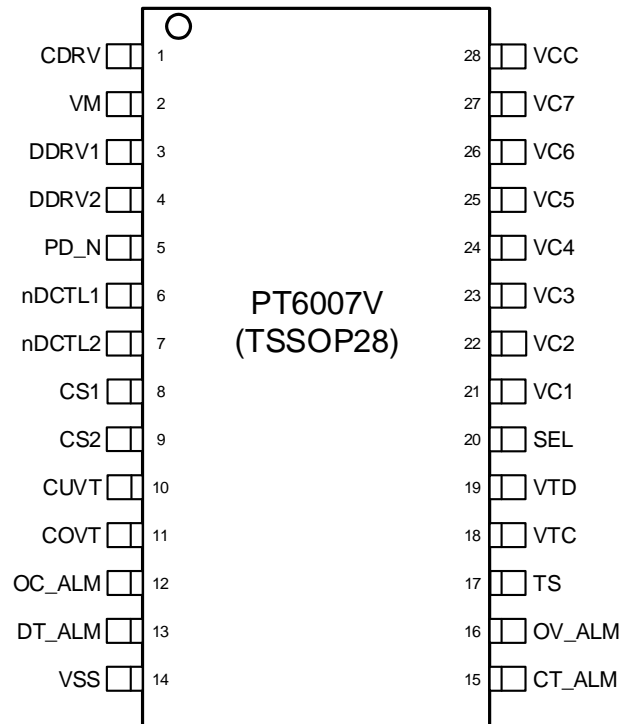
图 3. 管脚定义图
