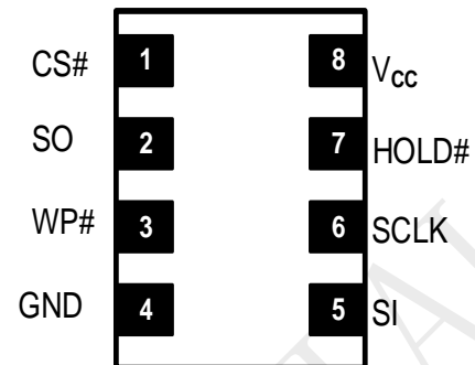
8-Land USON (3x2 / 1.5x1.5mm)
