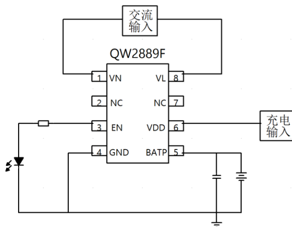
图一 QW2889F 典型应用电路
