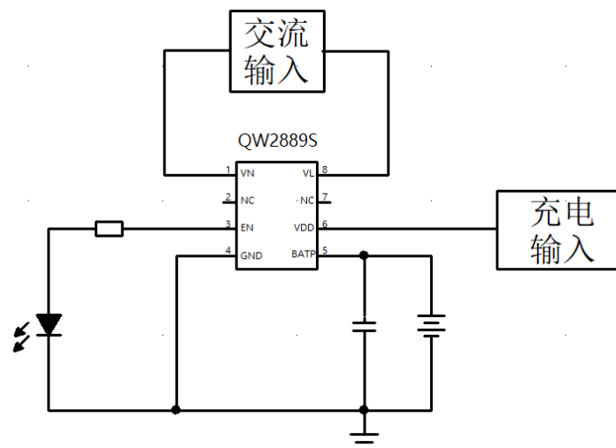
图一 QW2889S 典型应用电路
