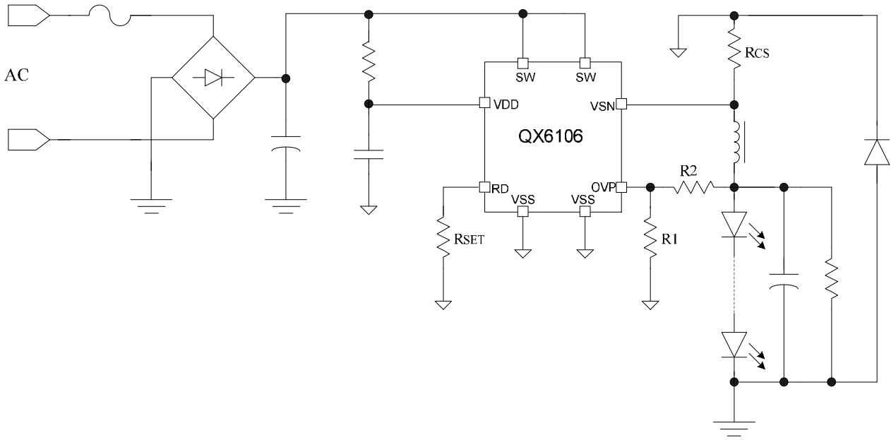
图 2: QX6106 典型应用电路图 2 (带输出电容)
