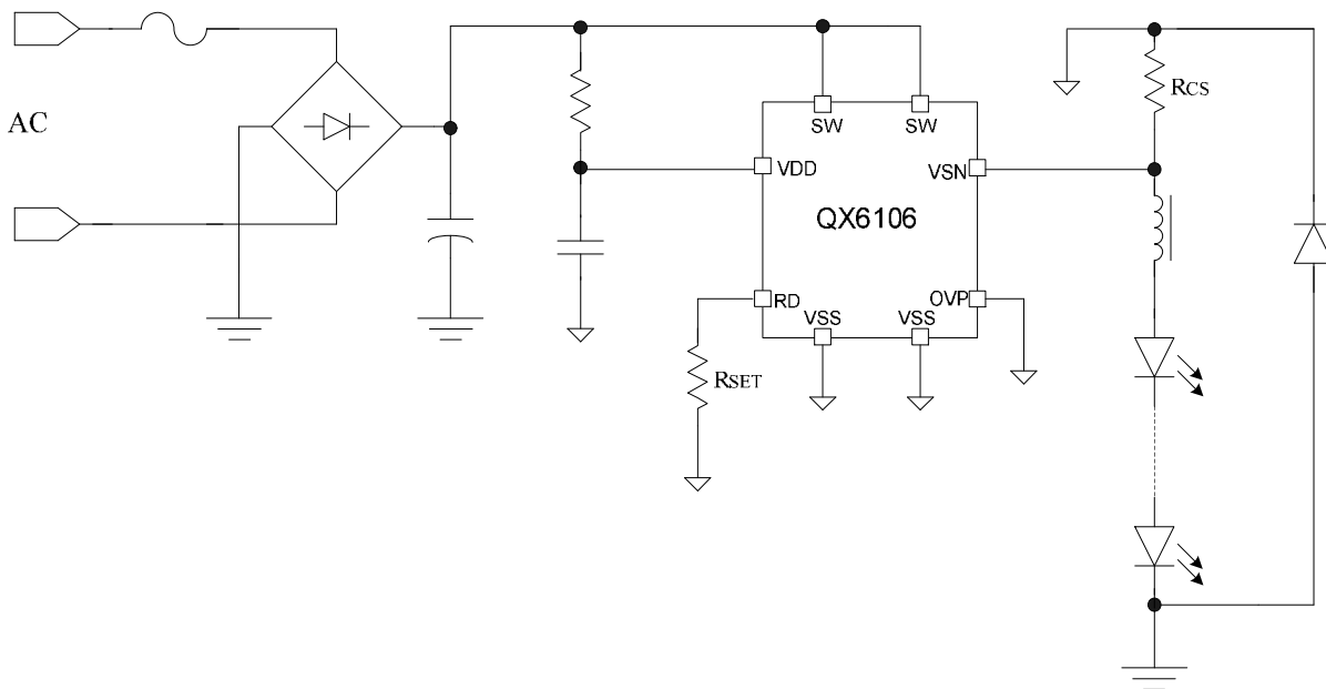
图 1: QX6106 典型应用电路图 1 (无输出电容)
