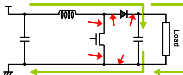
Fig. 2 MOSFET-OFF
