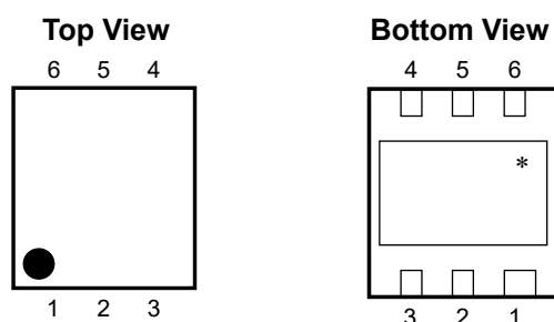
DFN(PL)1820-6
