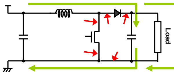
Fig. 2 MOSFET-OFF
