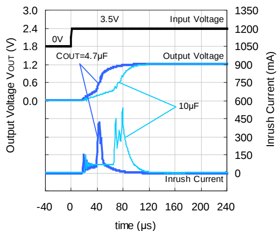
R1513S501B/D
