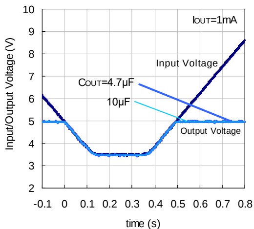
R1513S501B/D
