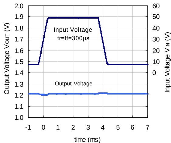
R1513S121B/D
