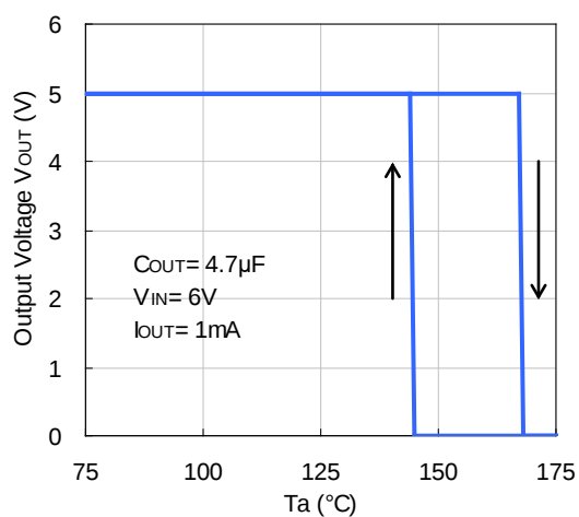
R1513S501B/D
