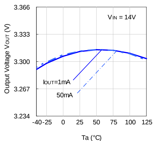
R1513S121B/D
