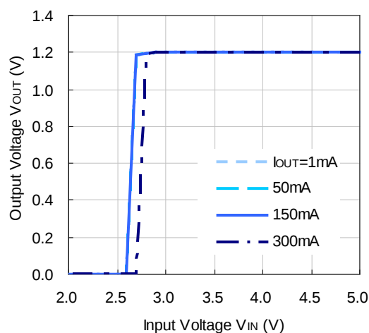
R1513S121B/D
