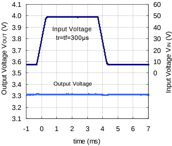
R1513S331B/D
