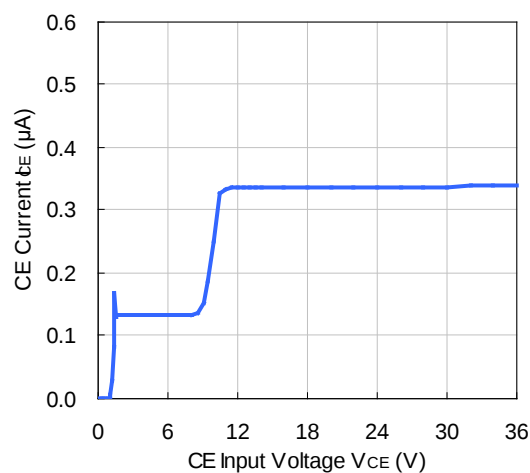
R1513Sxx1B/D
