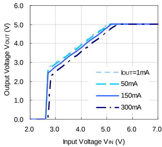
R1513S501B/D
