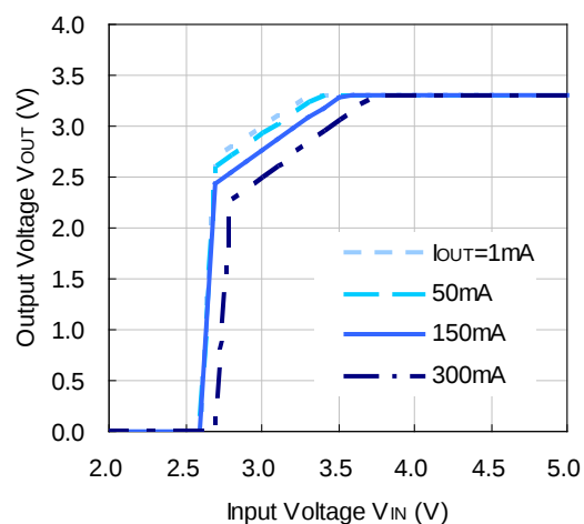
R1513S331B/D
