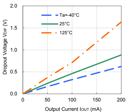
R8160x033B
