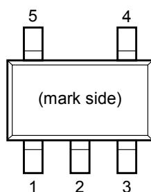
SOT-23-5
