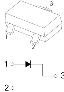
SOT-23
