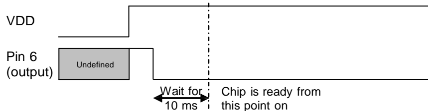
Figure 44. POR Timing Diagram
