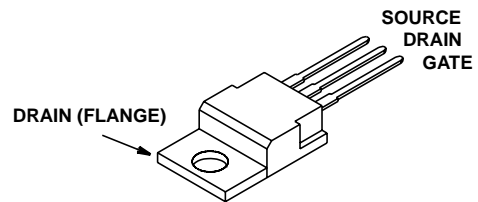
JEDEC TO-220AB
