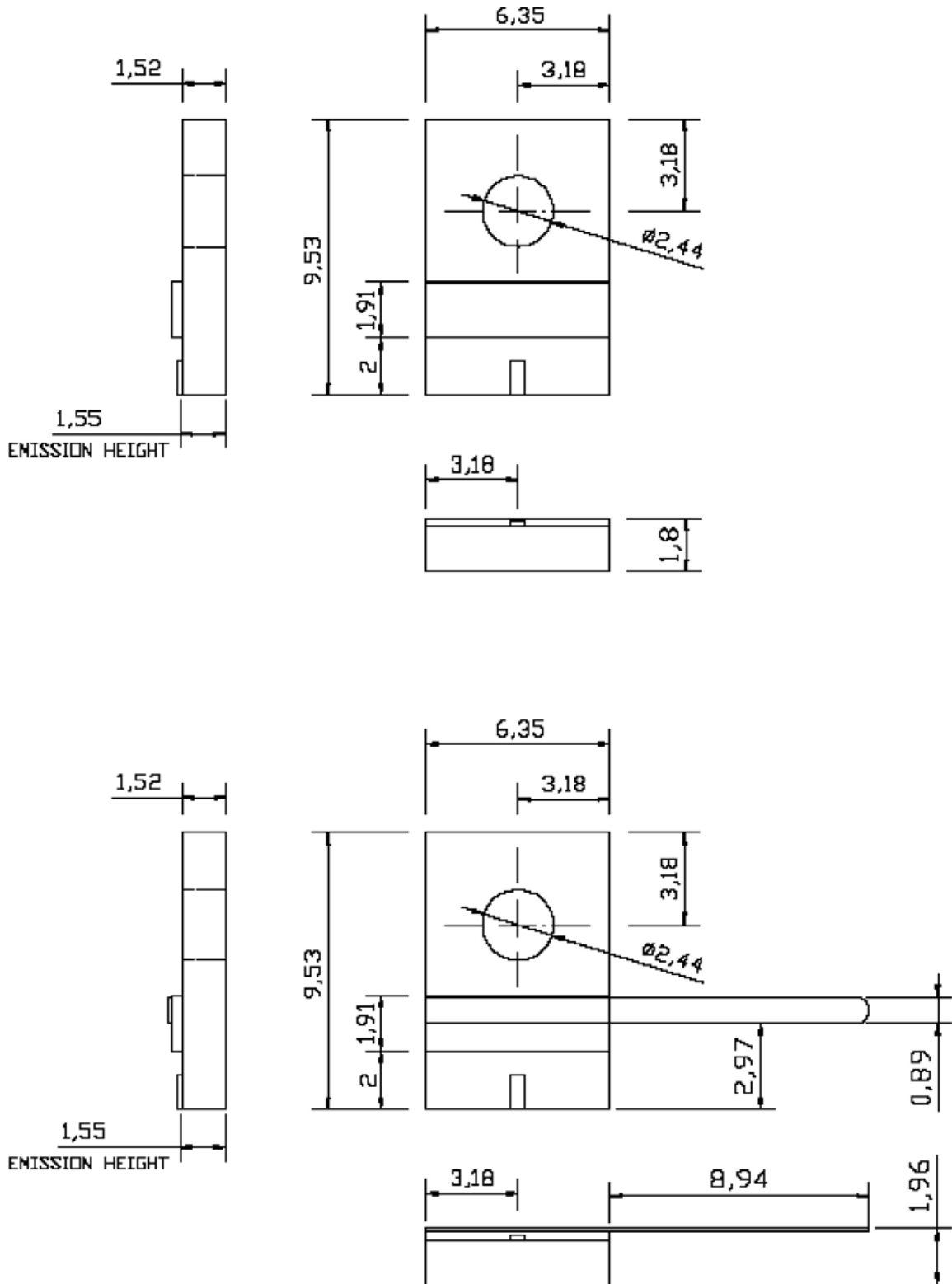
TO-3 Package (Unit:mm)
