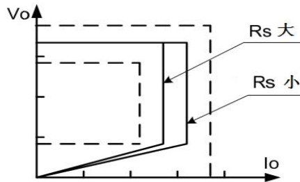
图3: 输出电流、功率与 R_s 关系曲线
