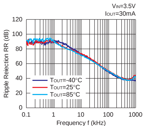
RP102x251x
