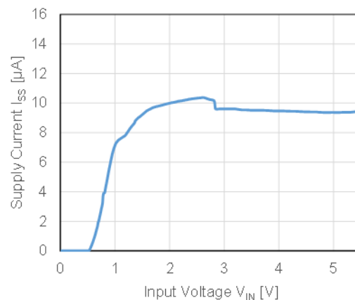
RP123x28xx
