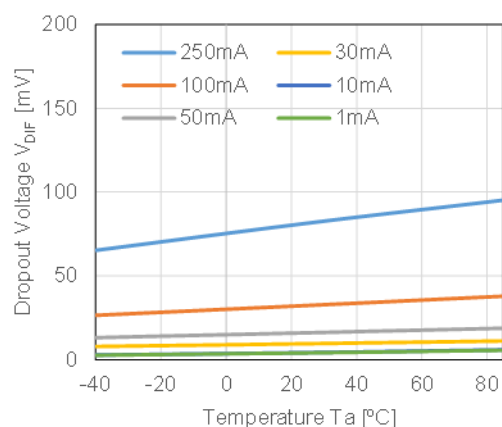
RP123Z28xx
