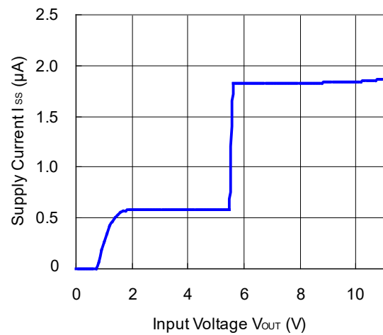
RP173x55xx
