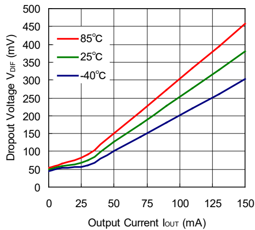
RP173x55xx
