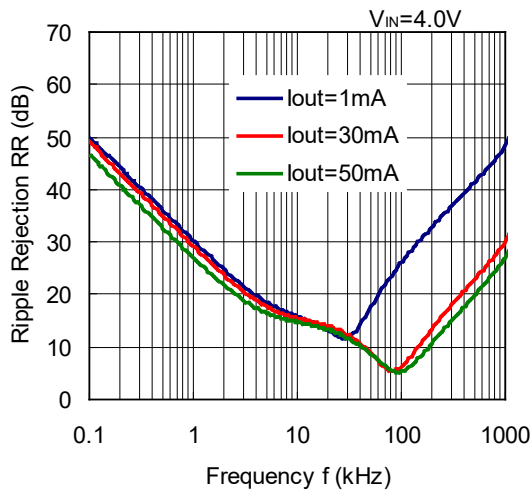
RP173x30xx
