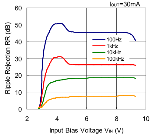
RP173x28xx
