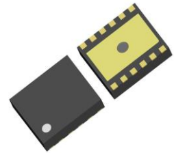
DFN(PL)2730-12 3.00 x 2.70 x 0.6
