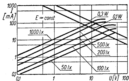
Charakterystyka prądowo-napięciowa fotorezystora RPP150
