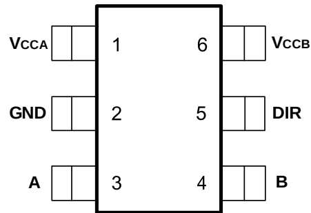
SOT23-6/SC70-6
