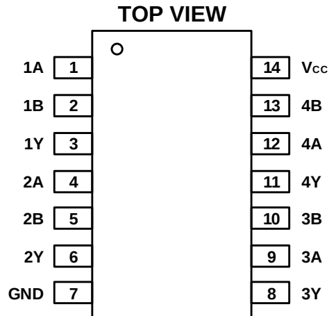
SOIC-14(SOP14)/TSSOP-14
