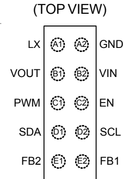
WL-CSP-10B 0.87x2.07(BSC)
