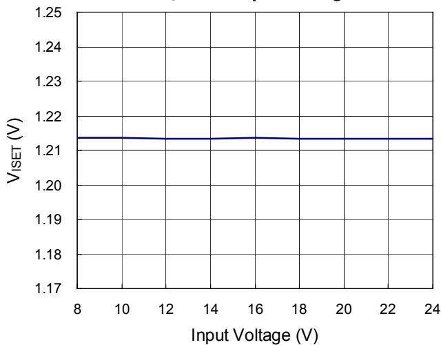
V_{ISET} vs. Input Voltage
