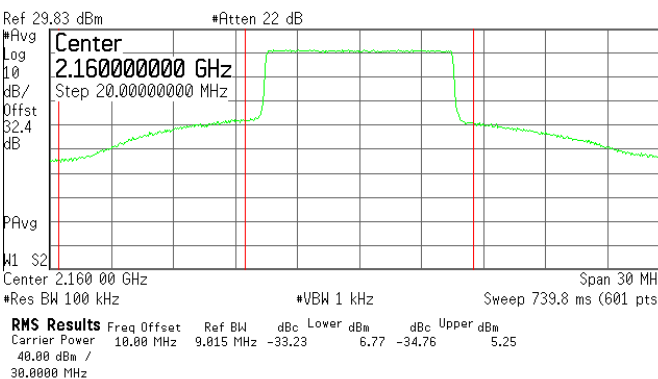
Pre - DPD@2160MHz
