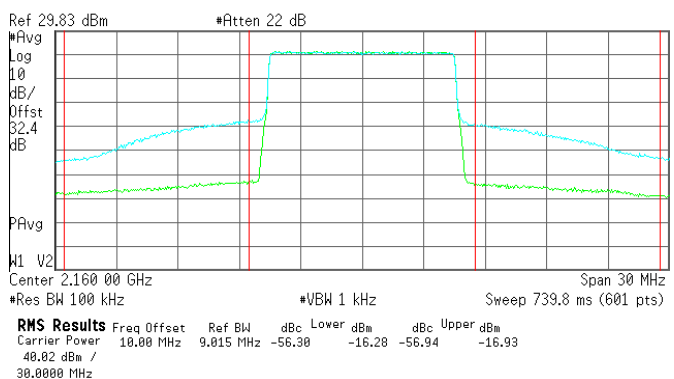
Post - DPD@2160MHz
