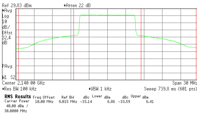
Pre - DPD@2140MHz
