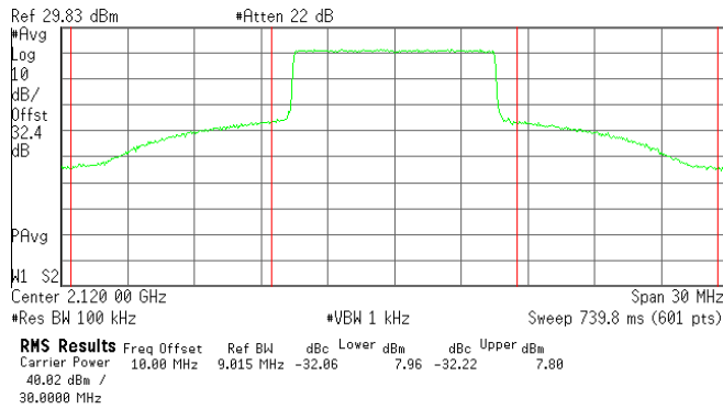
Pre - DPD@2120MHz
