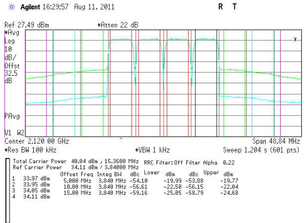
Post - DPD@2120MHz
