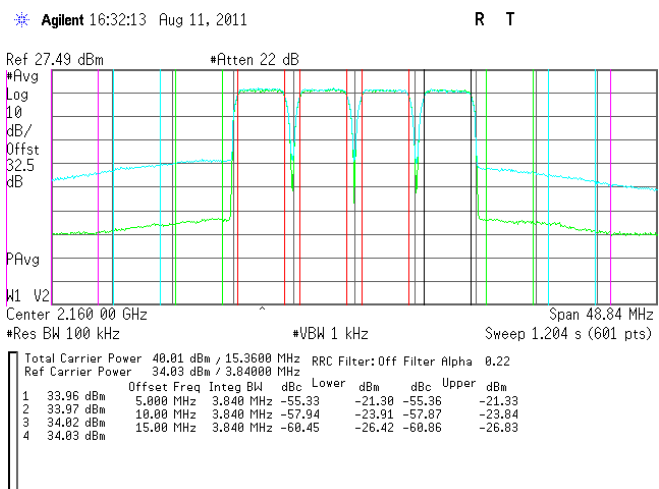
Post - DPD@2160MHz
