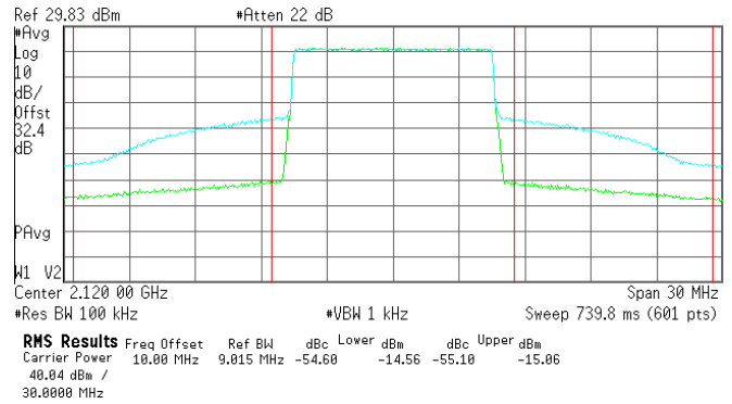
Post- DPD@2120MHz
