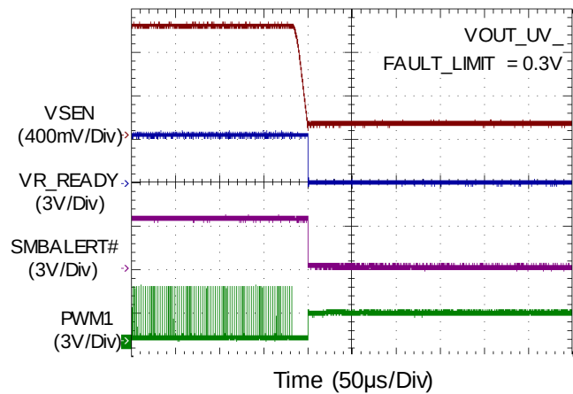
VR UVP
