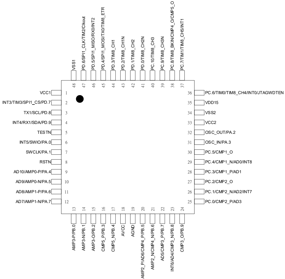
LQFP48
