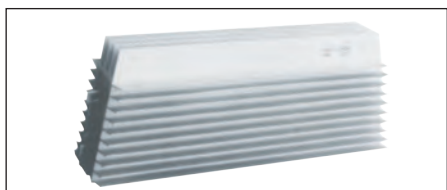
RXLG 铝合金电阻器 (带散热器 With heatsink) 功率：800W—1800W 阻值误差：±5%
