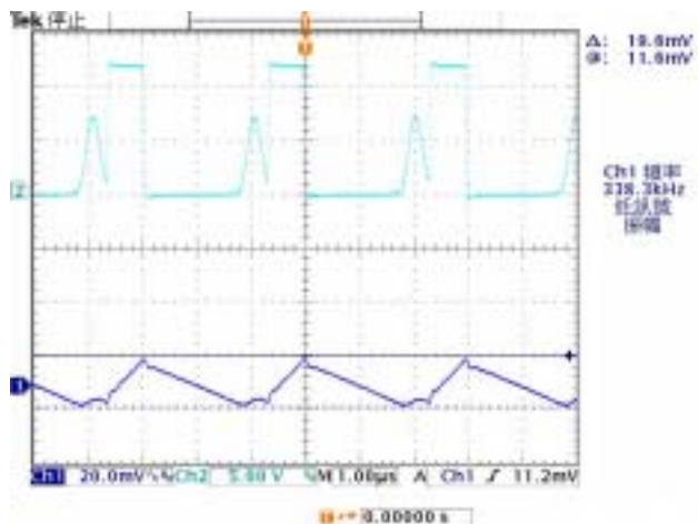
RZ1515 Vout Ripple (Vin=12V; Vout=3.3V; Iout=0.1A)
