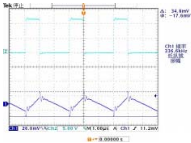
RZ1515 Vout Ripple (Vin=12V; Vout=3.3V; Iout=3A)
