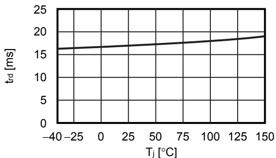
2. 6. 1 -V_{DET} = 2.6 V
