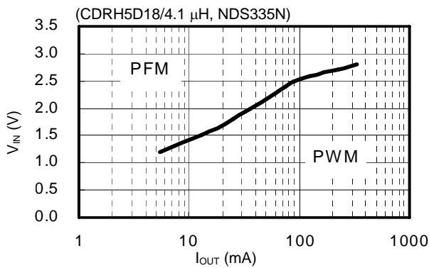
(29) S-8341A50AFT
