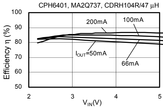
(24) S-8460B00AFT ( V_{OUT} = 3.3\text{ V} )
