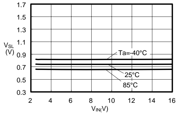
(8) V_{SL}-V_{IN}
