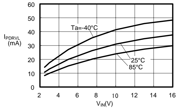
(4) I_{PDRVL}-V_{IN}
