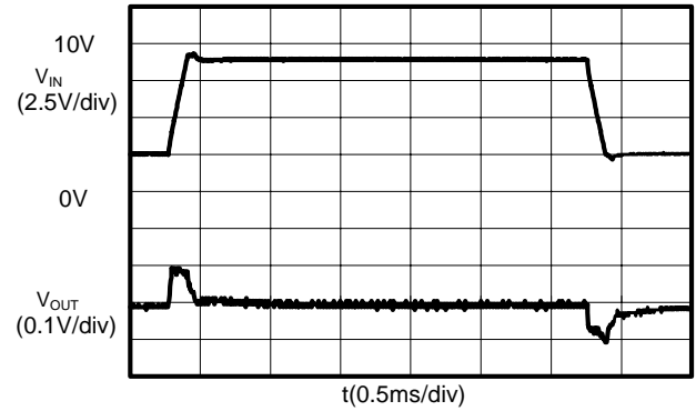
(2) S-8532B15AFT ( I_{OUT} : 500mA)
