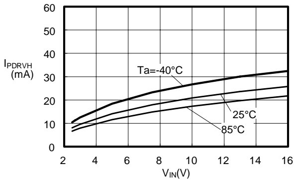
(3) I_{PDRVH}-V_{IN}
