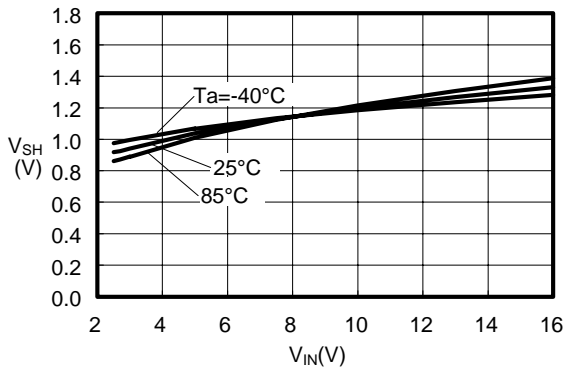
(7) V_{SH}-V_{IN}
