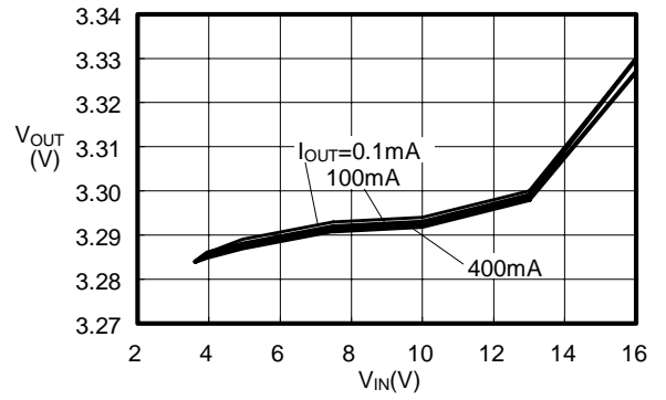
(11) V_{OUT}-V_{IN}
