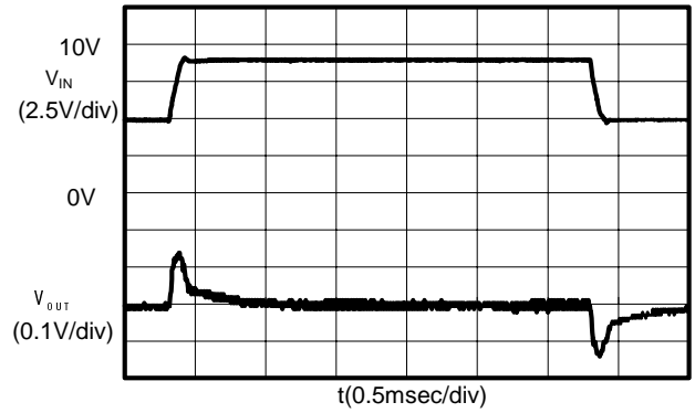
(4) S-8532B33AFT ( I_{OUT} : 500mA)
