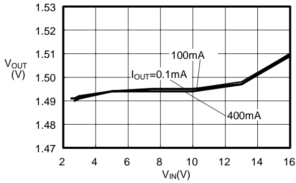
(10) V_{OUT}-V_{IN}
