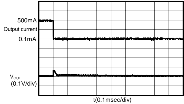
(2) S-8532B15AFT ( V_{IN} : 2.7V)
