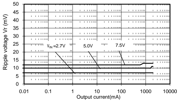
(29)S-8532B15AFT
