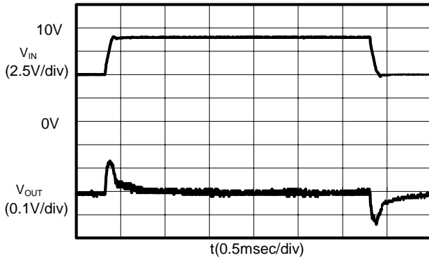
(3) S-8532B33AFT ( I_{OUT} : 10mA)
