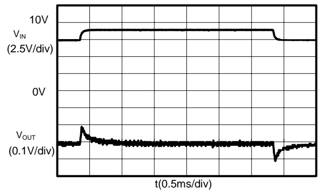
(6) S-8532B50AFT ( I_{OUT} : 500mA)
