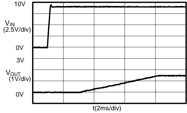
(2) S-8532B15AFT ( V_{IN} : 0→9.0V)
