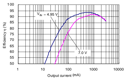
(25) S-8533A33AFT (CPH6303/CPH6403)
