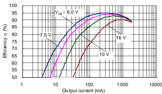
(15) S-8533A50AFT (CPH6302/CPH6402)
