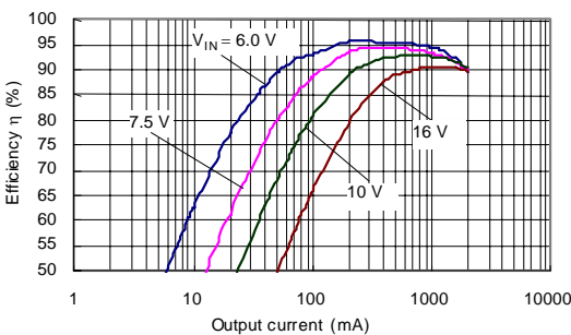
(23) S-8533A50AFT (CPH6302/CPH6402)
