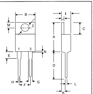
TO-220A
