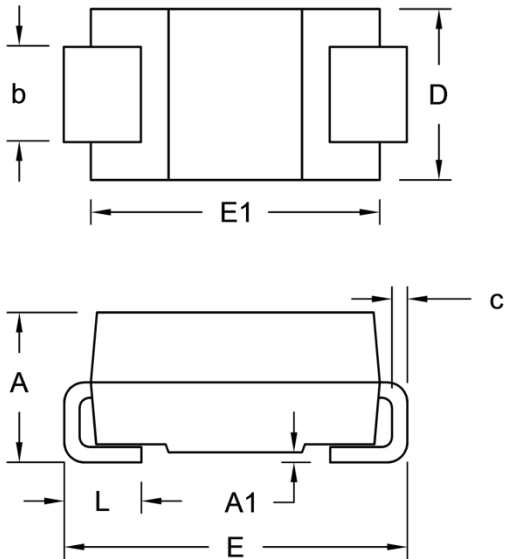
DO-214AC (SMA)
