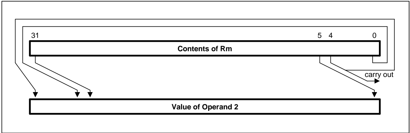
Figure 3-9. Rotate Right
