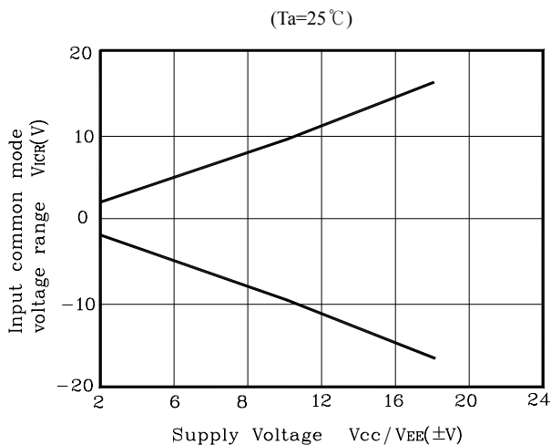
Fig. 4 V_{ICR} - V_{CC}/V_{EE}
