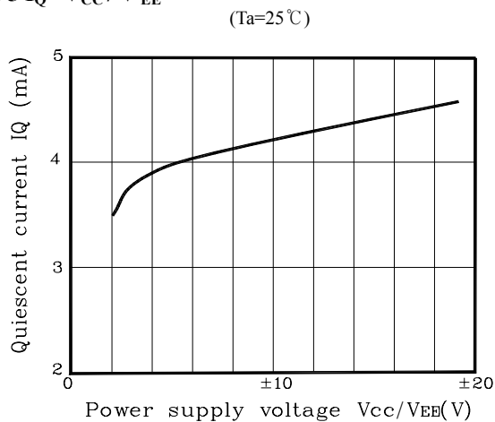
Fig. 5 I_Q - V_{CC}/V_{EE}
