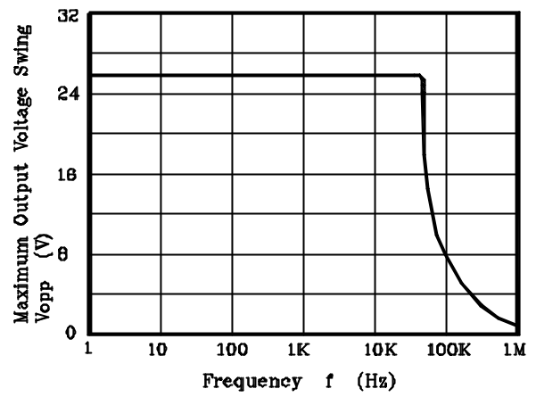
Fig. 2 V_{OP-P} - f
